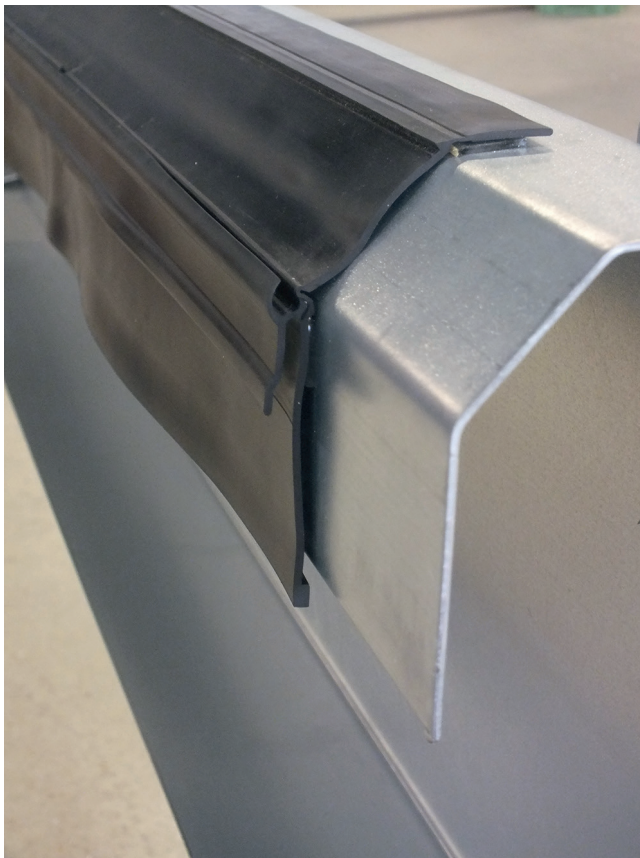
Zargensicherheitsanschluss ZSA Lichtband LB plus im Detail
