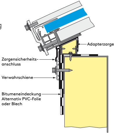
Zargensicherheitsanschluss ZSA Lichtband LB basic und LB plus mit Adapterzarge
