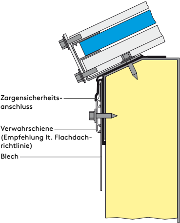
Zargensicherheitsanschluss ZSA Lichtband LB basic oder LB plus mit Blech-Dacheindeckung
