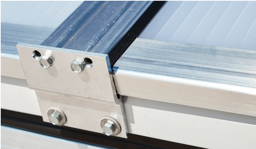
Zargensicherheitsanschluss ZSA am Lichtband LB plus
