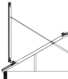
Einzel-Firstklappe mit NRWG- und Lüftungsklappensystem FlatFlap pneumatisch 30°
