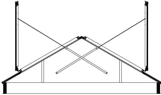
Doppel-Firstklappe mit NRWG- und Lüftungsklappensystem FlatFlap pneumatisch 30°
