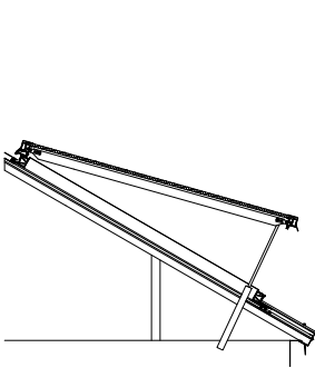
Einzel-Firstklappe mit Lüftungsklappensystem
