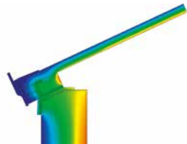
Isothermenverlauf Sattellichtband SLB plus im Querschnitt mit zusätzlicher Dämmung im Auflagebereich
