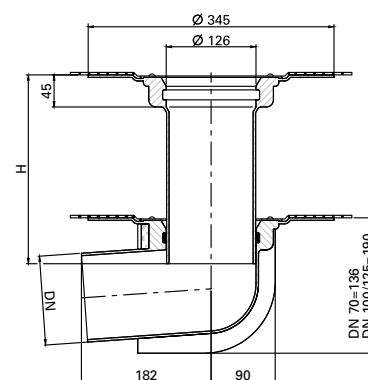
DN 70-125 Abgewinkelte Ausführung
