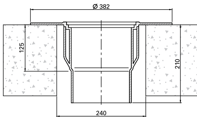
DN 150 senkrecht
