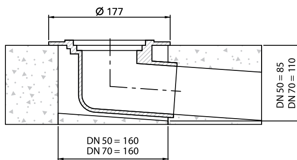
Balkongully Typ A abgewinkelt
