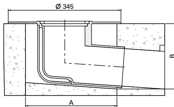
Dachgully abgewinkelt
