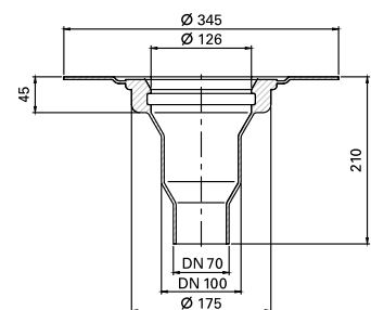
Kingspan ESSMANN Stufengully Ausführung Schraubflansch
