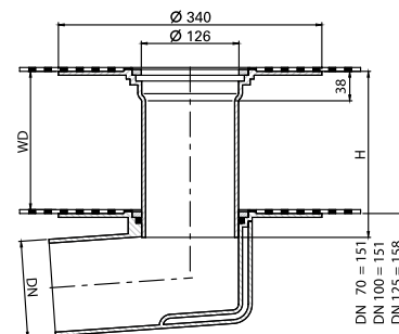
DN 70-125* Abgewinkelte Ausführung
