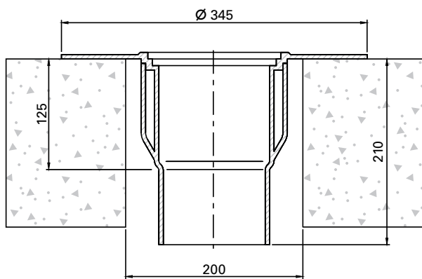
DN 70-125 senkrecht
