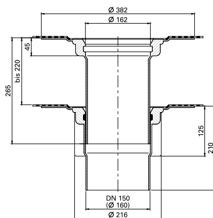
DN 150 Senkrechte Ausführung
