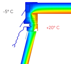
Optimierter Isothermenverlauf Dunkelklappe LK DKL neo plus für ein minimiertes Tauwasser- und Schimmelrisiko
