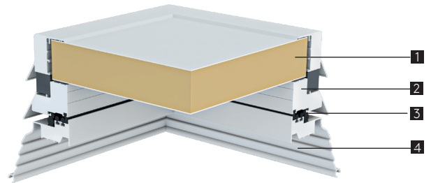
Dunkelklappe LK DKL neo plus mit Sandwichelement in 60 mm Stärke mit XPS Dämmung und Aluminiumdeckschicht im Querschnitt
