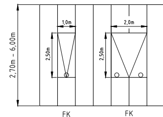
Klappenvarianten für Lichtband LB plus
