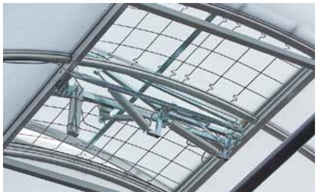
Lichtband LB plus mit Firstklappe, NRWG F6 LB und Ab- und Durchsturzsicherung EAD – Ansicht von unten
