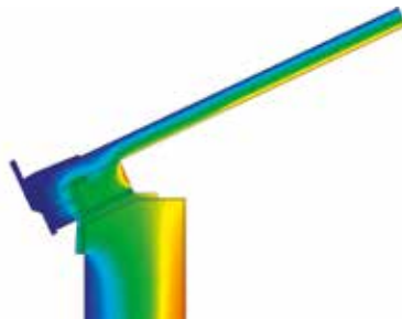
Isothermenverlauf Lichtband LB plus im Querschnitt mit zusätzlicher Dämmung im Auflagebereich
