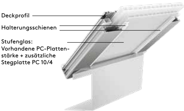
ERUglaz mit PC-Stegplatte 16/7 + 10/4 – im Querschnitt
