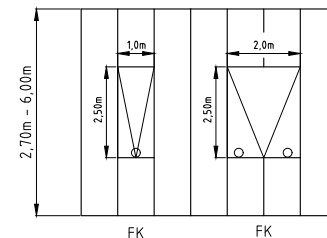
Klappenvarianten für Lichtband LB basic
