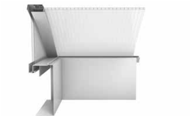
Lichtband LB basic im Schnitt – Frontalansicht
