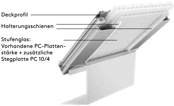
ERUglaz mit PC-Stegplatte 16/7 + 10/4 – im Querschnitt
