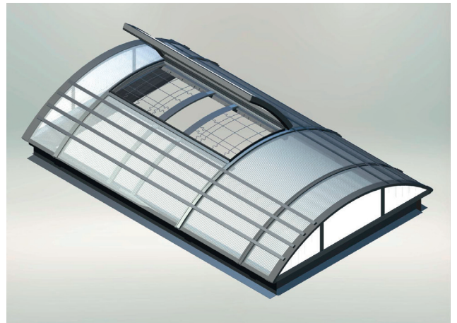
Lichtband LB plus mit integrierter Durchsturzsischerung ID 600, Ab- und Durchsturzsischerung EAD LB und 2 m Firstklappe, Ausführung für NRW
