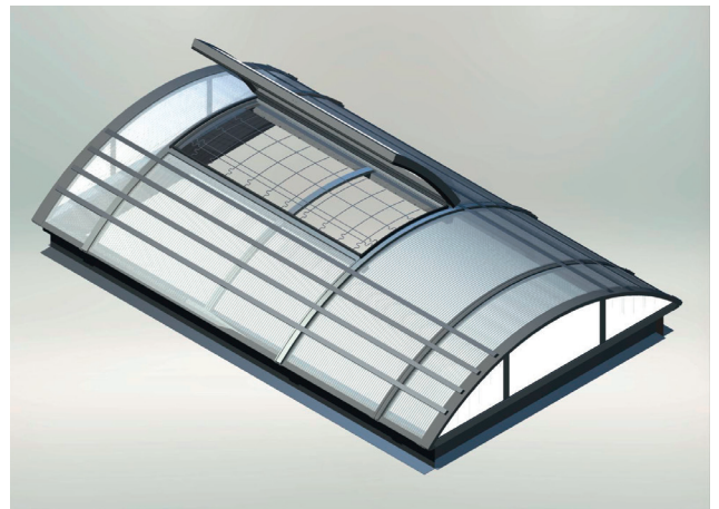
Lichtband LB plus mit integrierter Durchsturzsicherung ID 600, Ab- und Durchsturzsicherung EAD LB und 2 m Firstklappe mit Lüftungsfunktion
