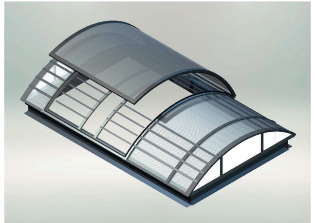
Lichtband LB plus mit integrierter Durchsturzsischerung ID 600 und 2 m Vollklappe, Ausführung für NRW
