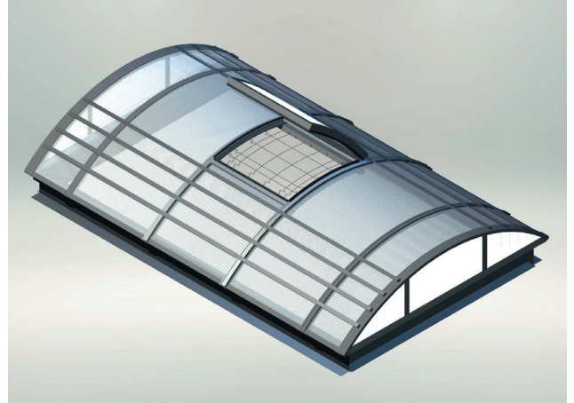
Lichtband LB plus mit integrierter Durchsturzsicherung ID 600, Ab- und Durchsturzsicherung EAD LB und 1 m Firstklappe mit Lüftungsfunktion
