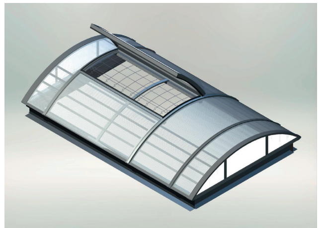
Lichtband LB plus mit integrierter Durchsturzsicherung ID 1200 plus, Ab- und Durchsturzsicherung EAD LB und 2 m Firstklappe mit Lüftungsfunktion
