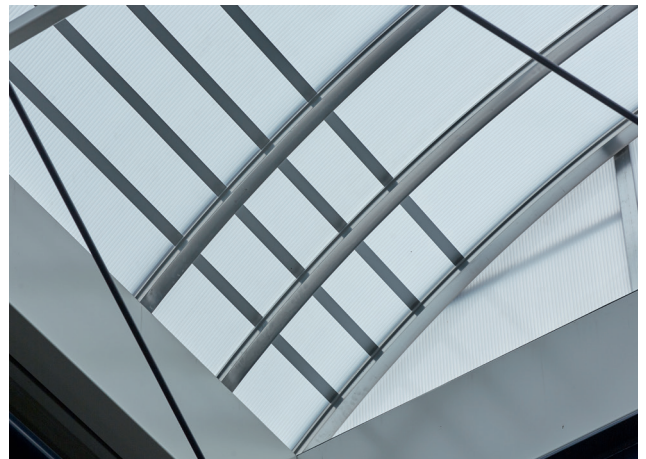
Lichtband LB plus mit integrierter Durchsturzsicherung ID 1200 plus im Detail – Ansicht von unten
