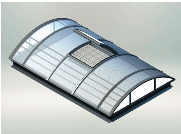
Lichtband LB plus mit integrierter Durchsturzsicherung ID 1200 plus, Ab- und Durchsturzsicherung EAD LB und 1 m Firstklappe mit Lüftungsfunktion
