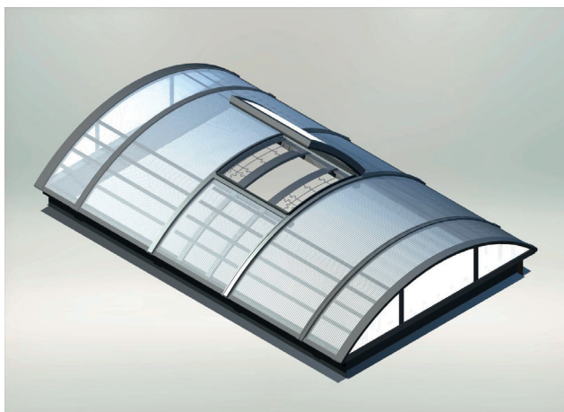
Lichtband LB plus mit integrierter Durchsturzsicherung ID 1200 plus, Ab- und Durchsturzsicherung EAD LB und 1 m Firstklappe, Ausführung für NRW
