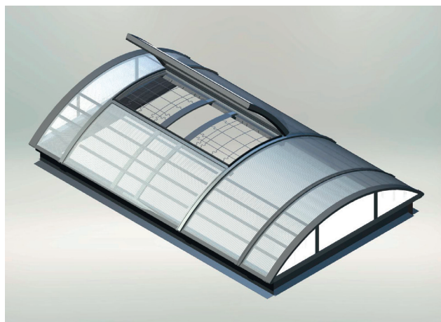
Lichtband LB plus mit integrierter Durchsturzsicherung ID 1200 plus, Ab- und Durchsturzsicherung EAD LB und 2 m Firstklappe, Ausführung für NRW
