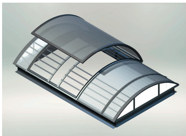
Lichtband LB plus mit integrierter Durchsturzsicherung ID 1200 plus und 2 m Vollklappe, Ausführung für NRW
