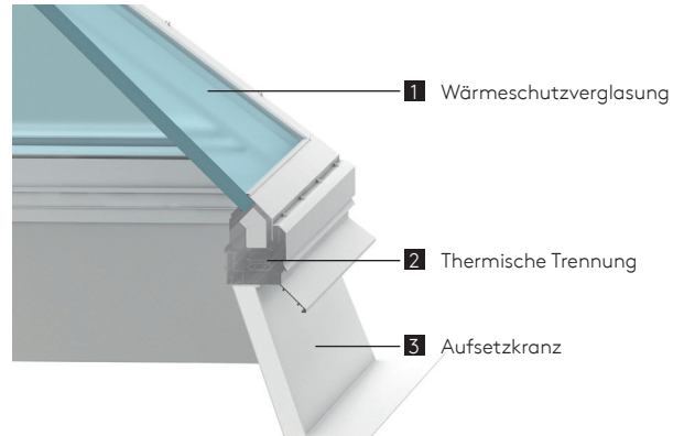
Glaspyramide GLP im Querschnitt
