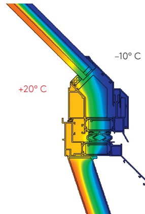
Isothermenverlauf Glaspyramide GLP
