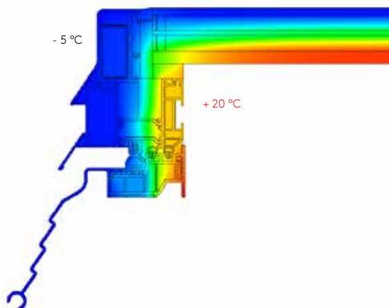
Isothermenverlauf Flachdachfenster neo mit 3-fach Wärmeschutzverglasung im Querschnitt
