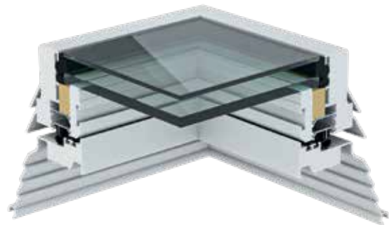
Flachdachfenster FDF neo mit 2-fach Wärmeschutzverglasung im Querschnitt
