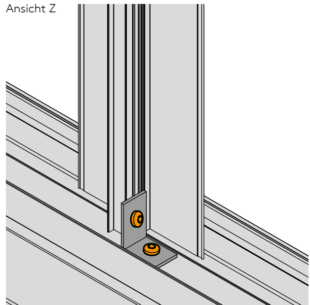
Ansicht Z
