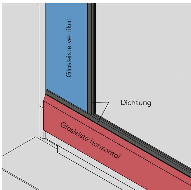
Ansicht Z
