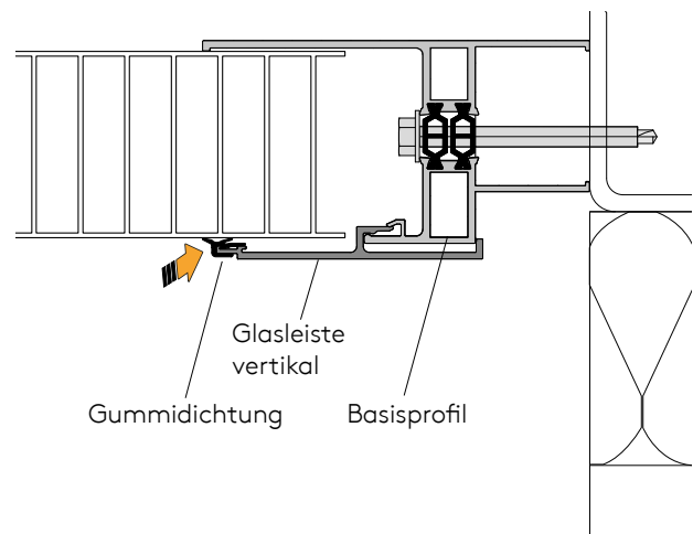
Ansicht B - B
