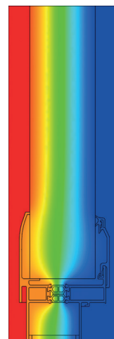
Isothermenverlauf Funktionsfassade Aurora mit PC 60/13 Verglasung
