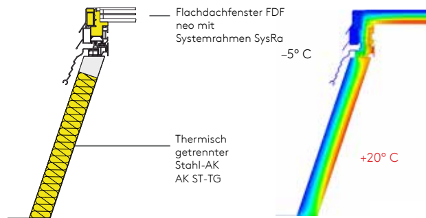
Links: Flachdachfenster FDF neo mit 3-fach Verglasung im Querschnitt und schrägem thermisch getrennten Stahl-Aufsetzkranz AK ST-TG Rechts: Isothermenverlauf Flachdachfenster FDF neo mit 3-fach Verglasung und schrägem thermisch getrennten Stahl-Aufsetzkranz AK ST-TG
